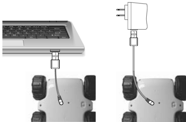
Первый способ зарядки
